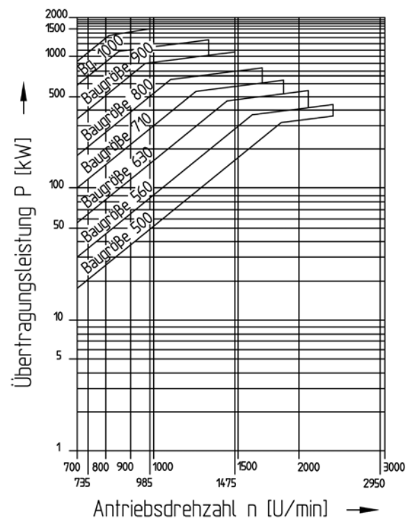
Leistungskennfeld doppelutige Ausführung (Außenradantrieb)
